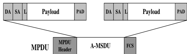
Fig.22 A-MSDU data
