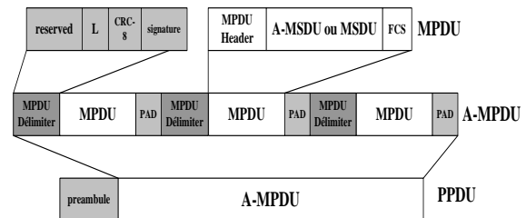
Fig.26 A-MPDU data
